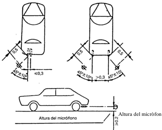
Figura 3. Posició de l'instrument de mesura en vehicles automòbils
