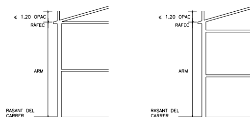
CROQUIS núm. 4 RAFEC DE L'EDIFICI
